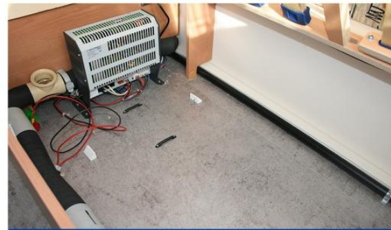
Stap 8: Plaats bepalen elektronica & accu
